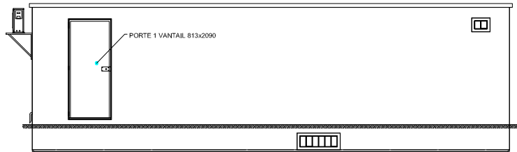
FACE ARRIERE
